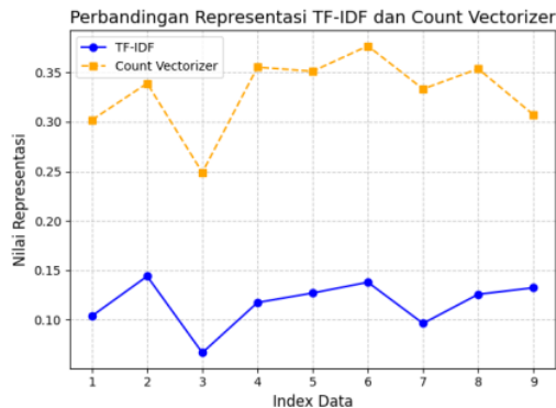
Gambar 2. Hasil Uji Skenario 1
