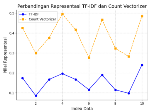
Gambar 3. Hasil Uji Skenario 2
