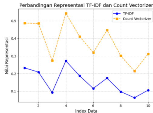
Gambar 4. Hasil Uji Skenario 3
